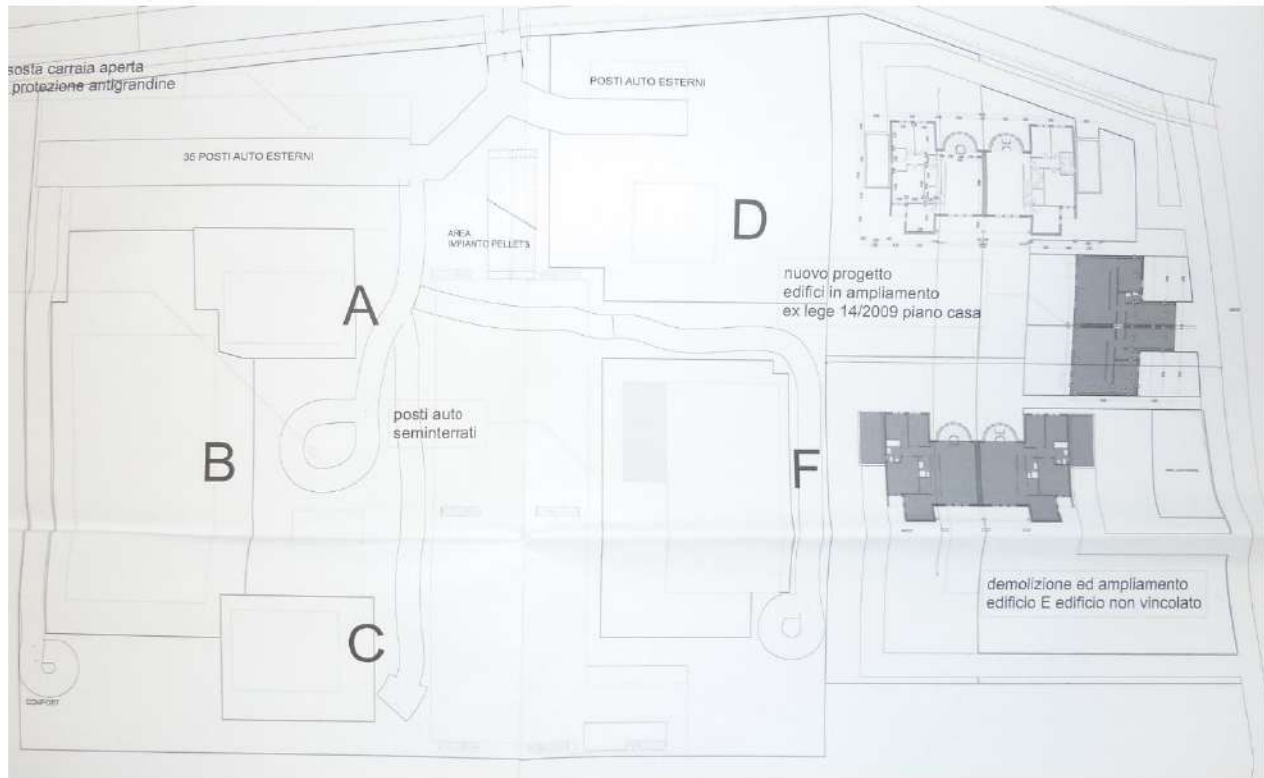
Schema planimetrico con piante dei fabbricati ed evidenziazione dei relativi lotti di pertinenza
